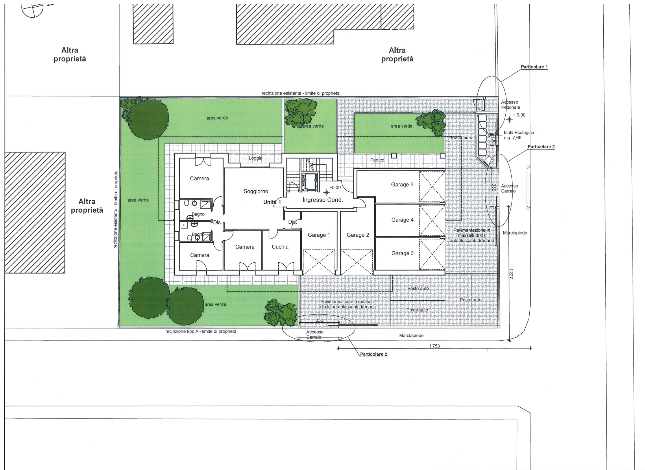
Planimetria con Sistemazioni esterne scala 1:200
